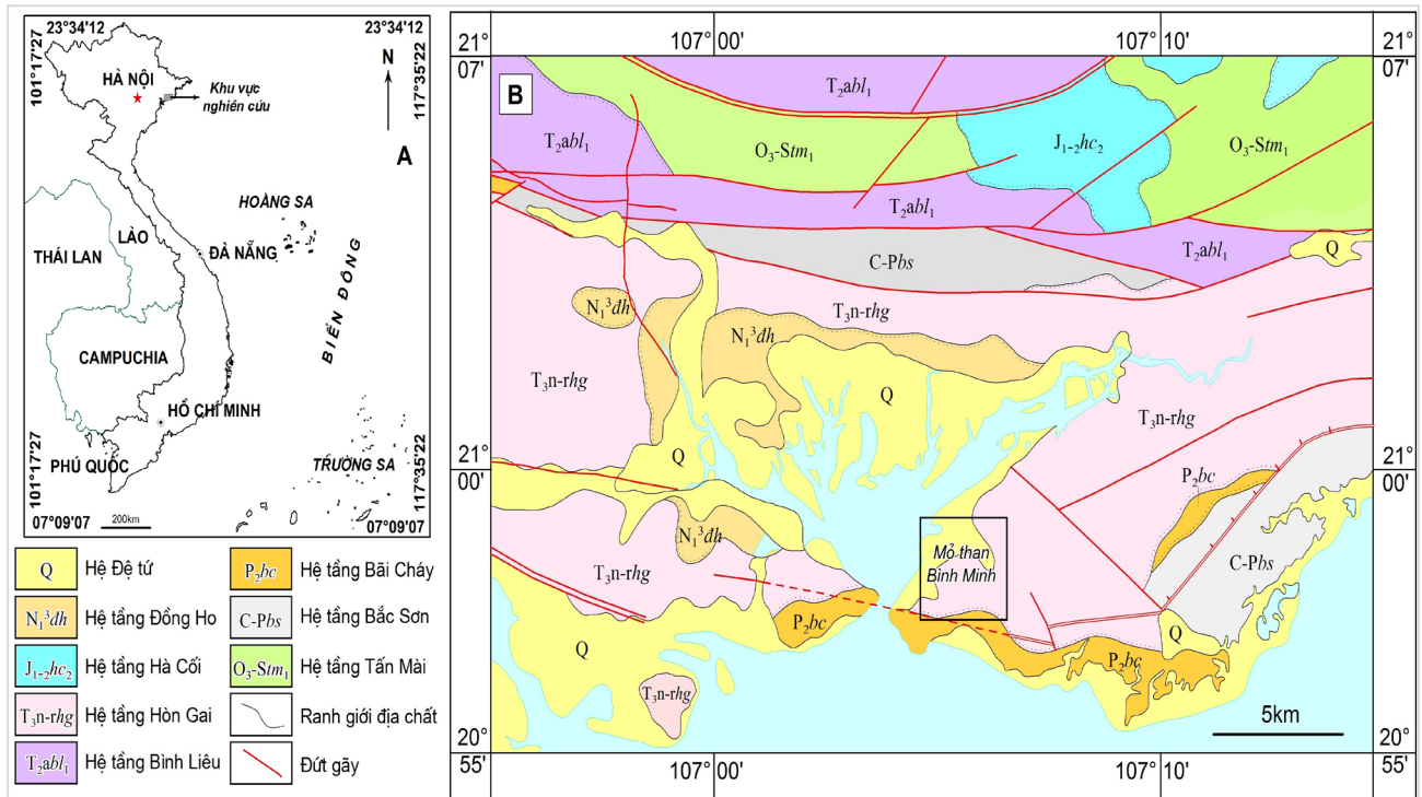
Hình 1. Sơ đồ Việt Nam và vị trí khu vực nghiên cứu (A); Sơ đồ địa chất khu mỏ than Bình Minh, tỉnh Quảng Ninh (Lê, 1996) (B).
